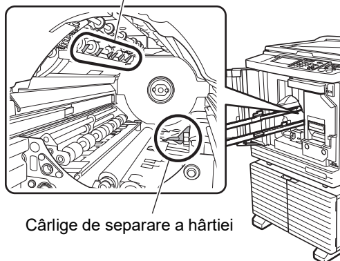
Cârlige de scoatere a matriței
