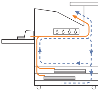
<스택 트레이를 사용할 경우>
